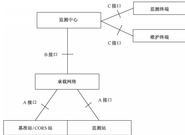
图1 监测系统组成示意图
