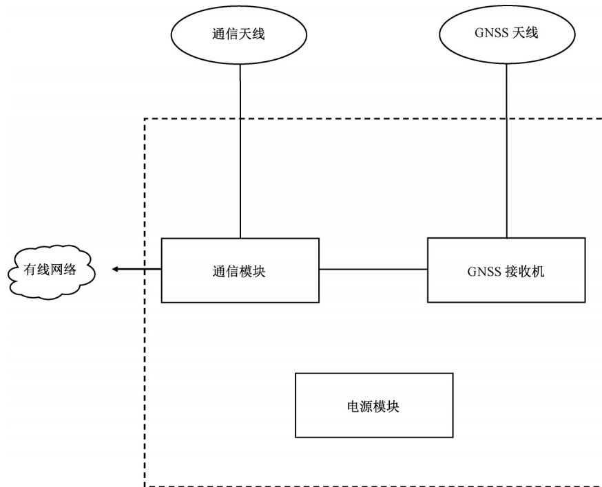
图3 监测站设备组成图
