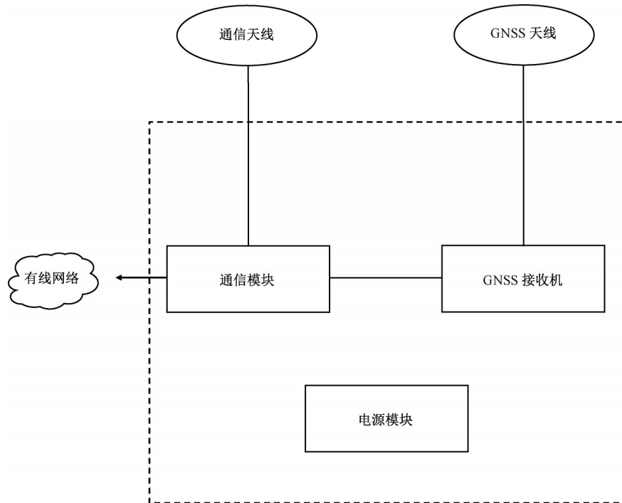
图2 基准站设备组成示意图
